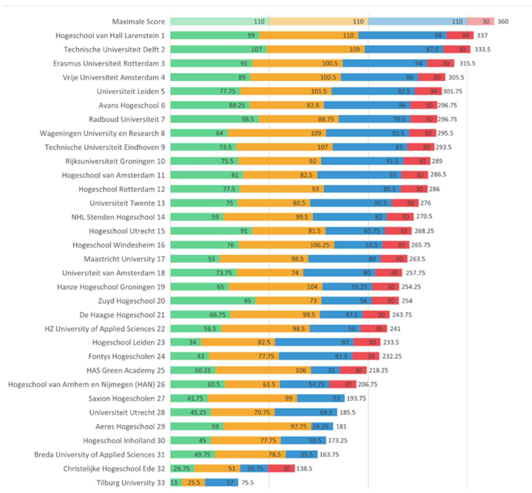
(圖表) SustainaBul 2024 荷蘭各校永續得分，綠色、橙色、藍色和紅色分別代表教育、研究、營運和最佳實踐各領域的分數。
