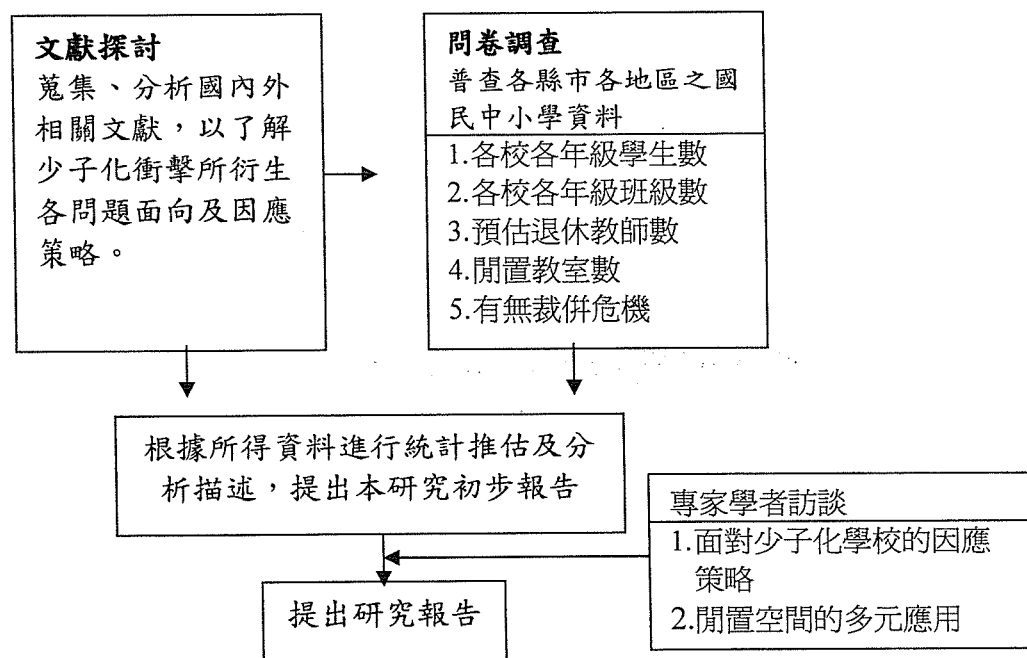
圖 3-1-1 研究架構圖
